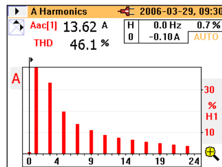
Figura 6. Gráfico de barras de armónicos de la corriente
