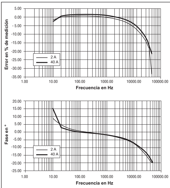
Figura 2. Respuesta de frecuencia a 2 y 40 A
