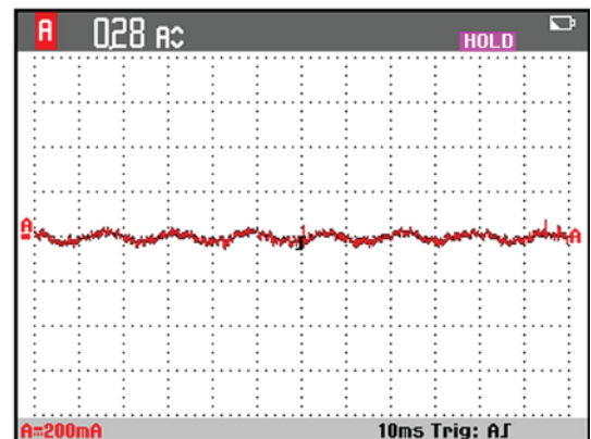
Figure 3. PE current.
