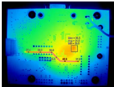
Tepelné vyhodnocování rozvržení desek s tištěnými spoji za účelem určení oblasti možných problémů
