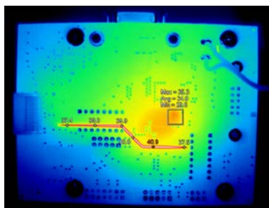
Evaluación térmica de zonas potencialmente problemáticas para el trazado de circuitos impresos
