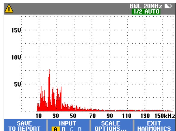
Spectre harmonique étendu de 9 kHz à 150 kHz
