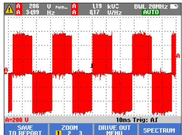
Forme d'onde de sortie du variateur de vitesse avec déclenchement automatique
