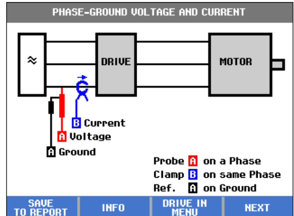
Raccordements de mesures guidées pas à pas de l'entrée du variateur de vitesse
