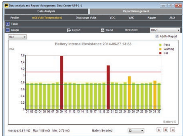
含使用者定義閾值的電池組直方圖。
