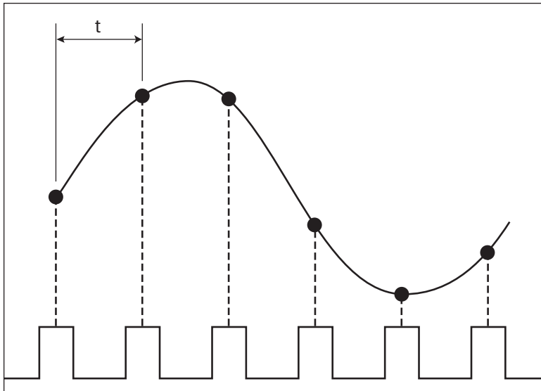
샘플링 및 보간: 샘플링은 점으로 표시되는 반면, 보간은 검은 선으로 표시됩니다.
