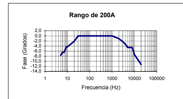
Figure 2. Desplazamiento de fase con respecto a frecuencia (Rango de 200A)
