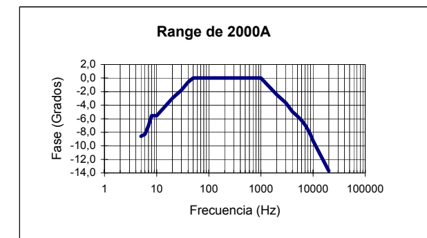
Figure 3. Desplazamiento de fase con respecto a frecuencia (Rango de 2000A)
