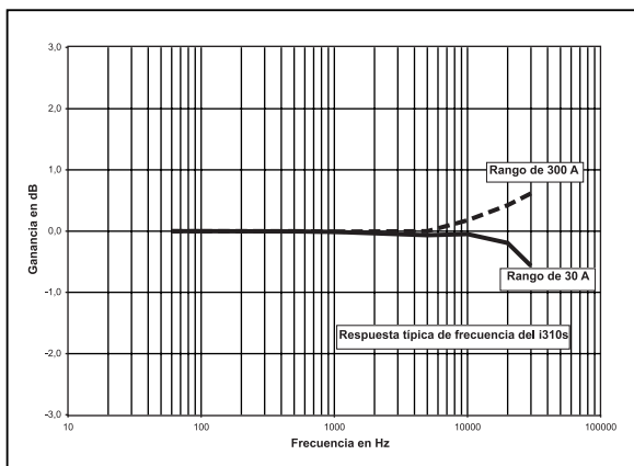
Respuesta típica de frecuencia
